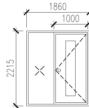
1x vstupní dveře, NE PLAST 1860x2215
